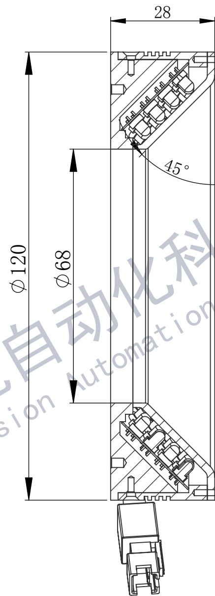
剖面 H-H
